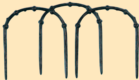
Rasenbegrenzung „Wien“ Art. 19401: B 600 mm x H 250 mm (Zierteilhöhe 100 mm, Erdspeiß 150 mm)
